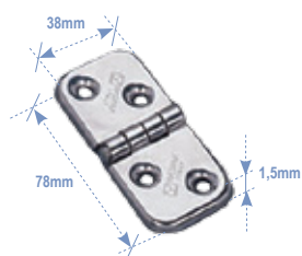
Hinge, Inox 316
