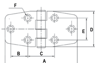
Hinge, Inox 316
